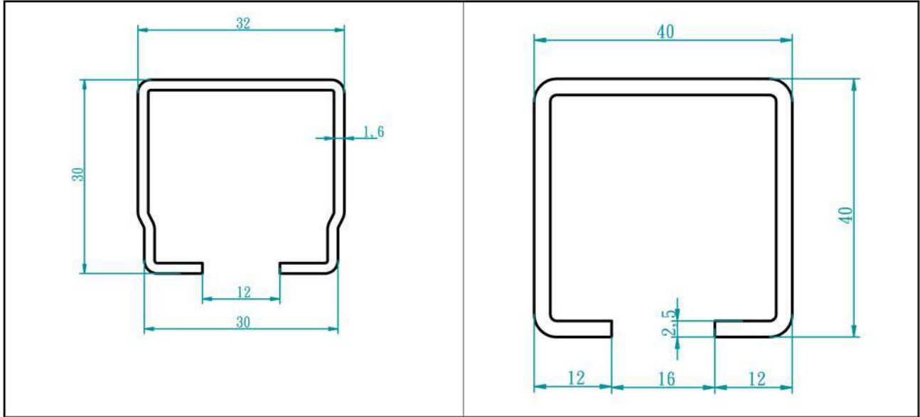
C30軌道斷面圖
